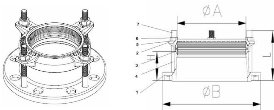
Рис.4. Муфта/адаптер ПФРК-Е
