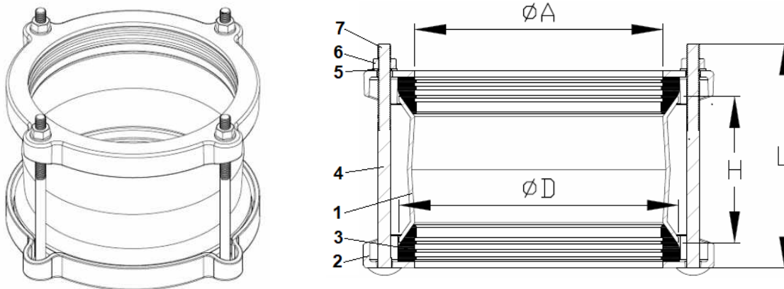
Рис.1. Муфта ДРК
